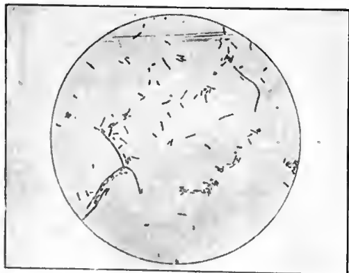
BACILLUS TYPHOSUS.
